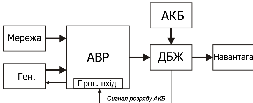
Рис. 5.9 – Блок-схема спільної роботи АВР та ДБЖ
