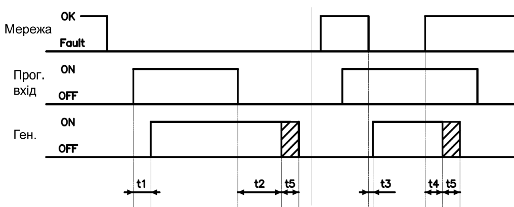
Рис. 5.10 – Діаграма роботи при виборі функції «Дозвіл запуску»
