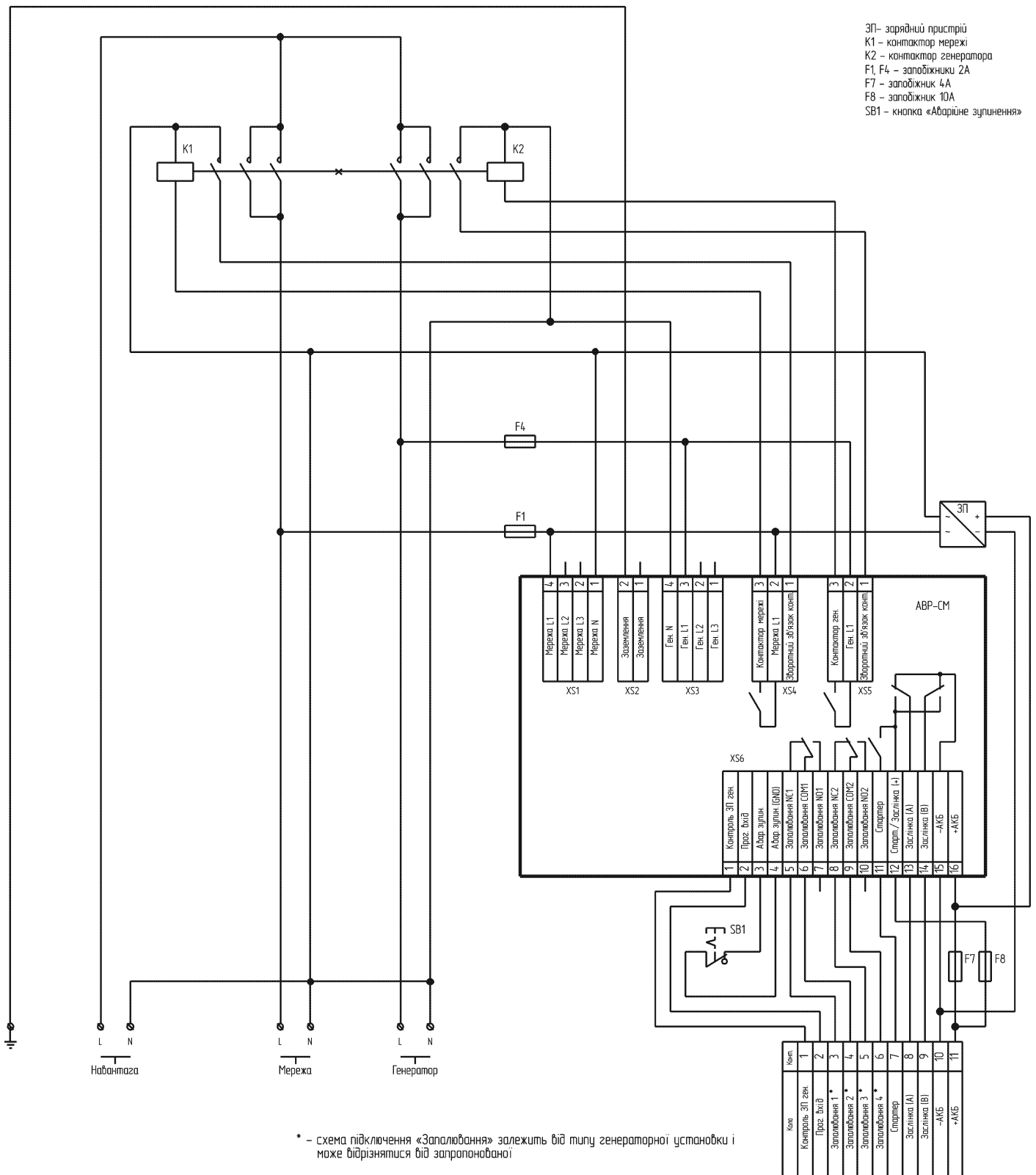
Рис. 6.4 – Схема підключення контролера для конфігурації AVR11 зі спільним нейтральним проводом
