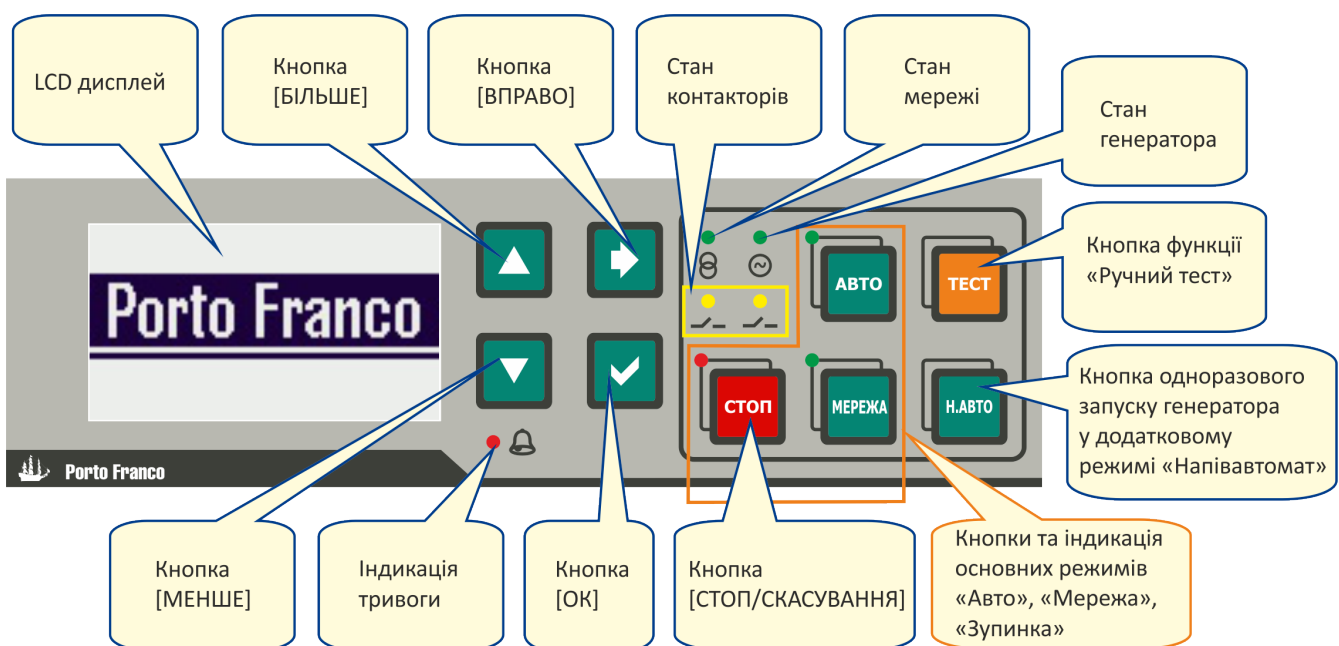
Рис. 5.2 – Панель індикації та управління
