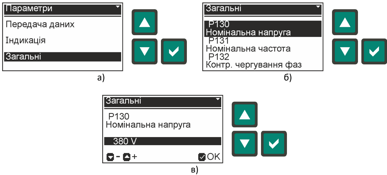
Рис. 5.14 – Приклад зміни параметра P130 – «Номінальна напруга»: а) вибір групи параметрів; б) вибір параметра; в) зміна параметра
