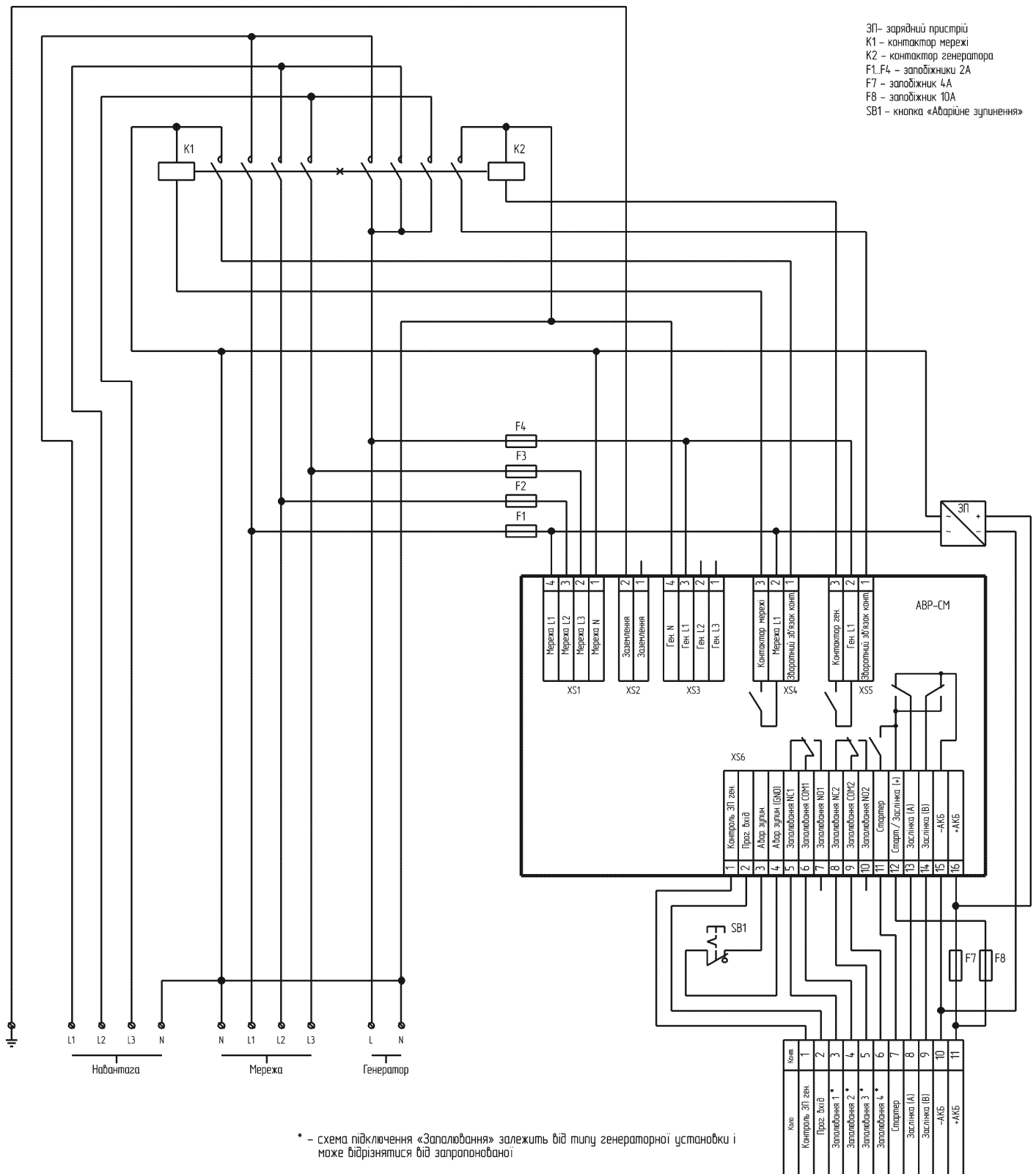
Рис. 6.3 – Схема підключення контролера для конфігурації AVR313 зі спільним нейтральним проводом
