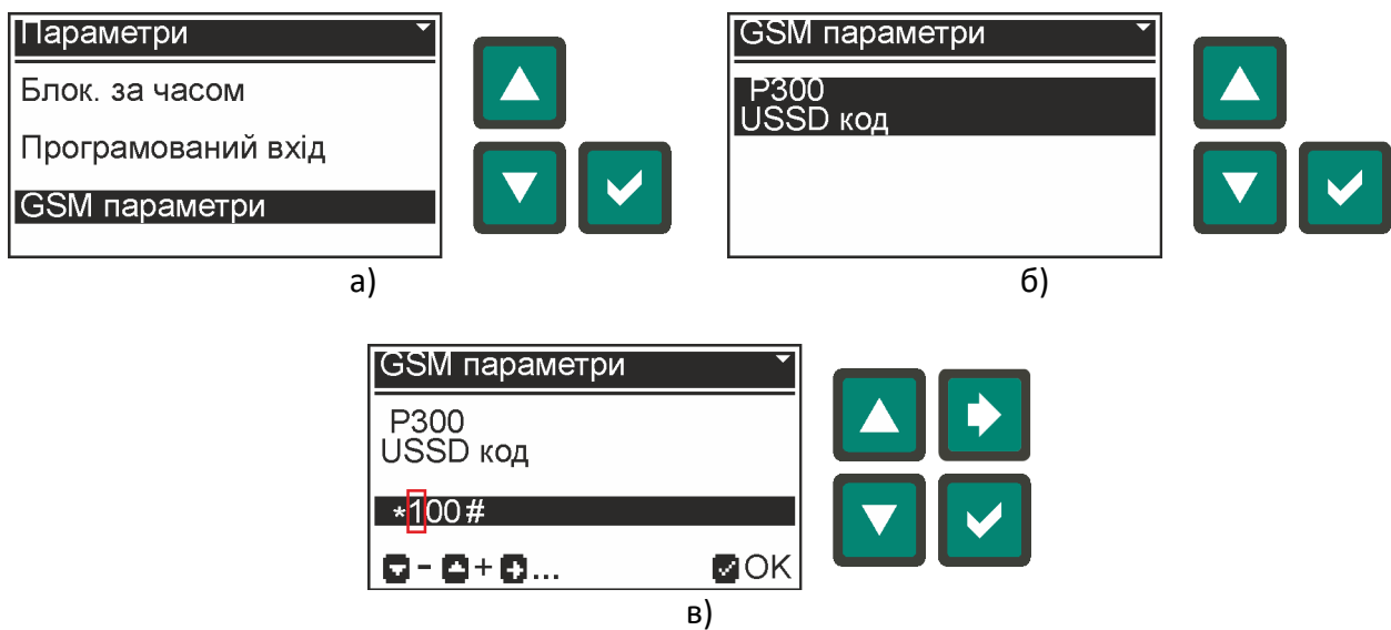
Рис. 5.15 – Приклад параметра P300 – «USSD код» з посимвольним редагуванням значення: а) вибір групи параметрів; б) вибір параметра; в) зміна параметра
