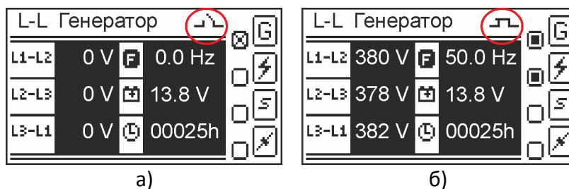
Рис. 5.8 – Індикація стану програмованого входу:
