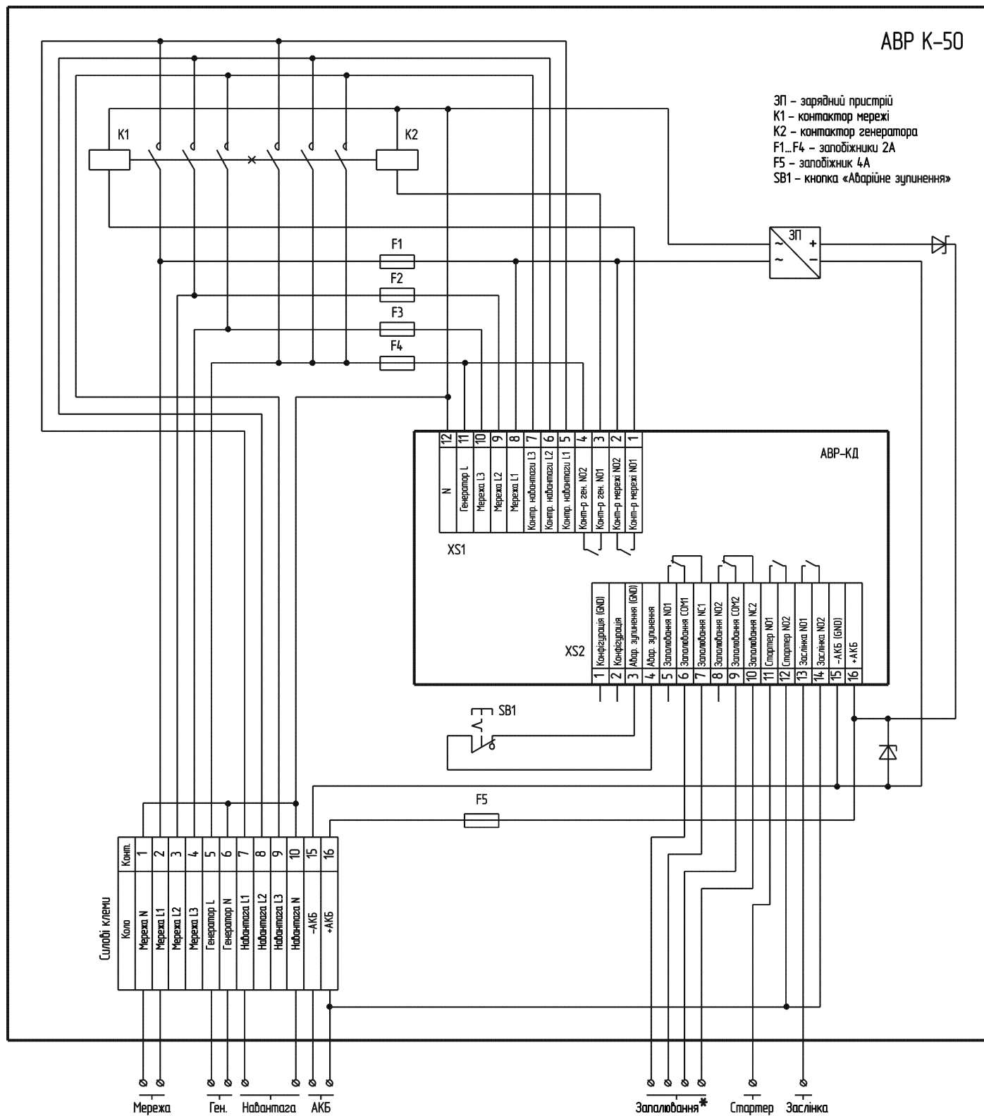
Рис. 6.4 – Приклад схеми підключення контролера ABP K-50 для однофазної мережі
